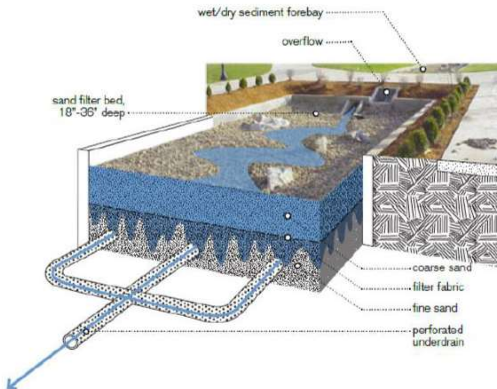
Figura 105. Schema tipo
