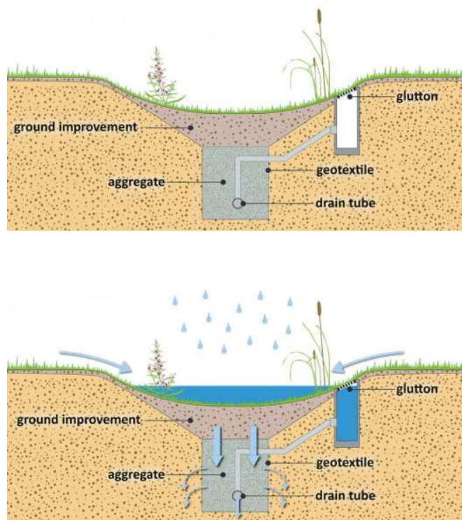
Figura 246. Schema tipo
