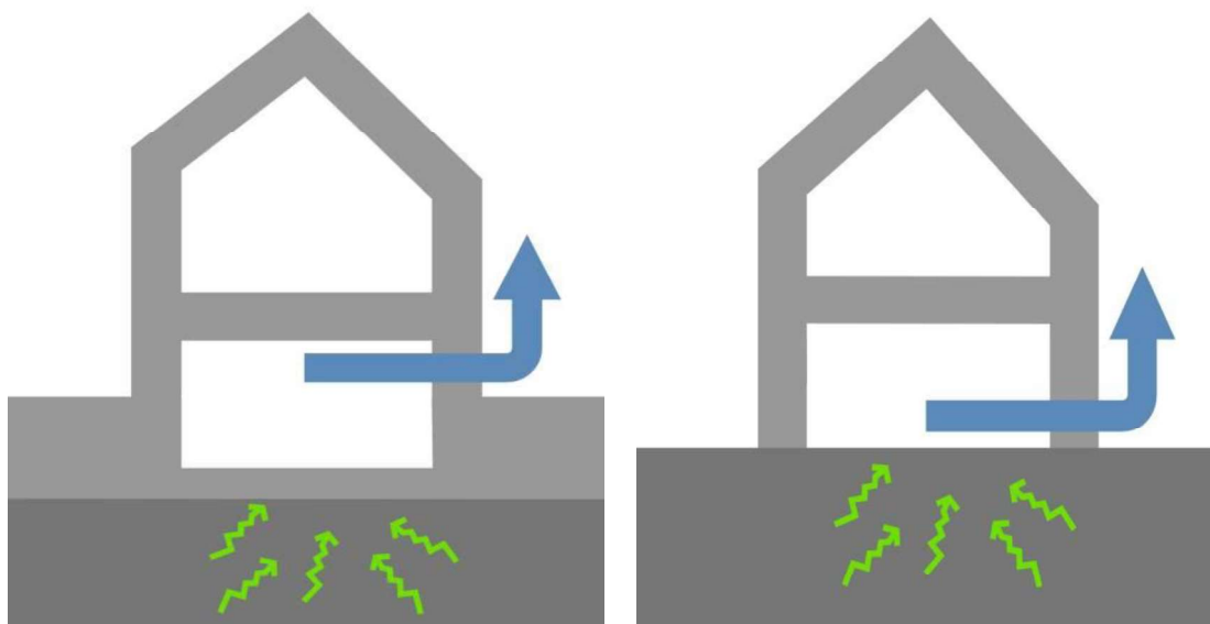
Figura 11: depressione di un volume tecnico sotto l'edificio
