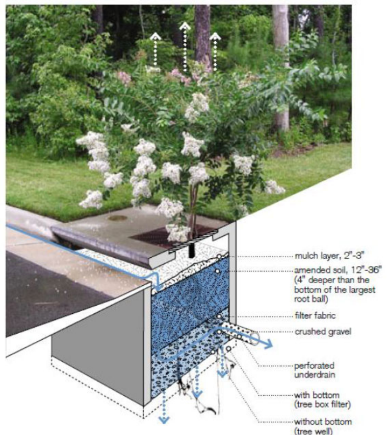
Figura 187. Schema tipo di Tree Box filter
