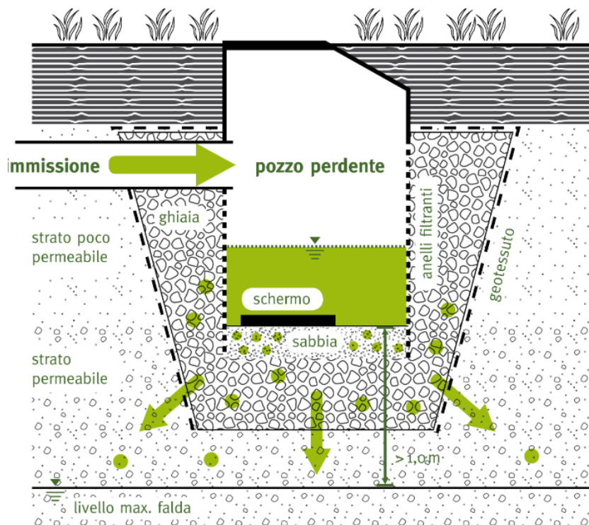
Figura 209. Schema tipo di realizzazione pozzo perdente
