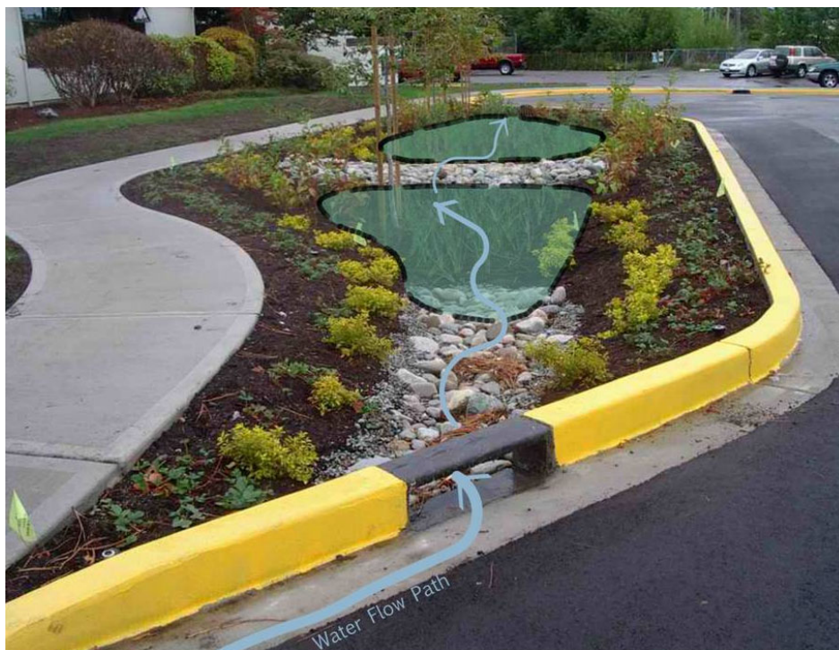
Figura 176. Rain Garden a servizio di lottizzazioni o privati
