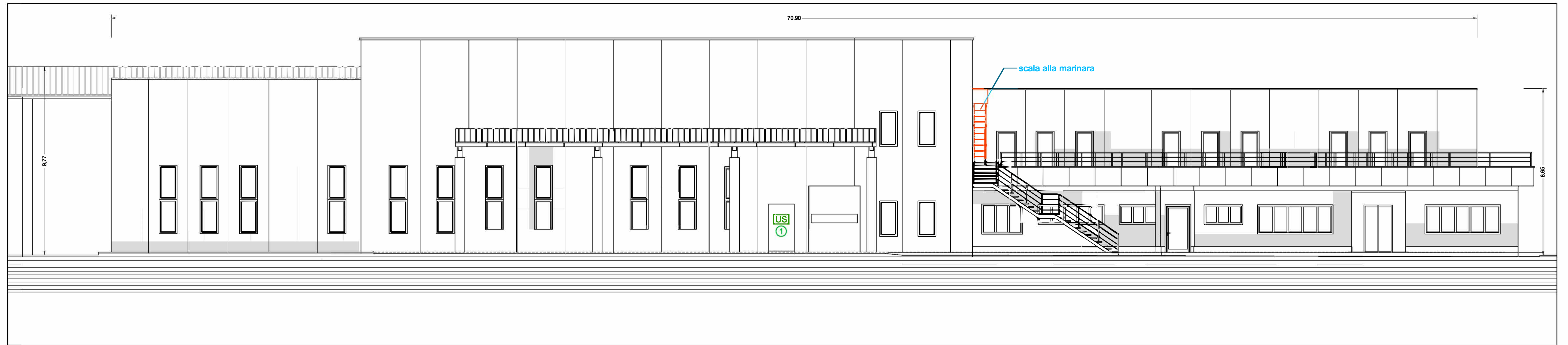
Prospetto VISTA 1 Scala 1:100
