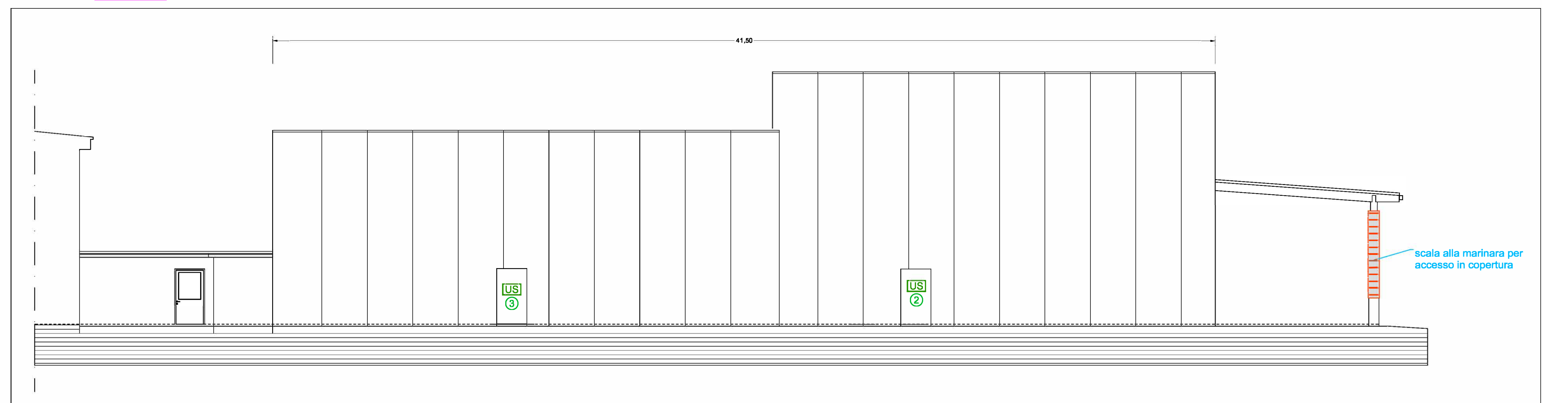
Prospetto VISTA 2 Scala 1:100
