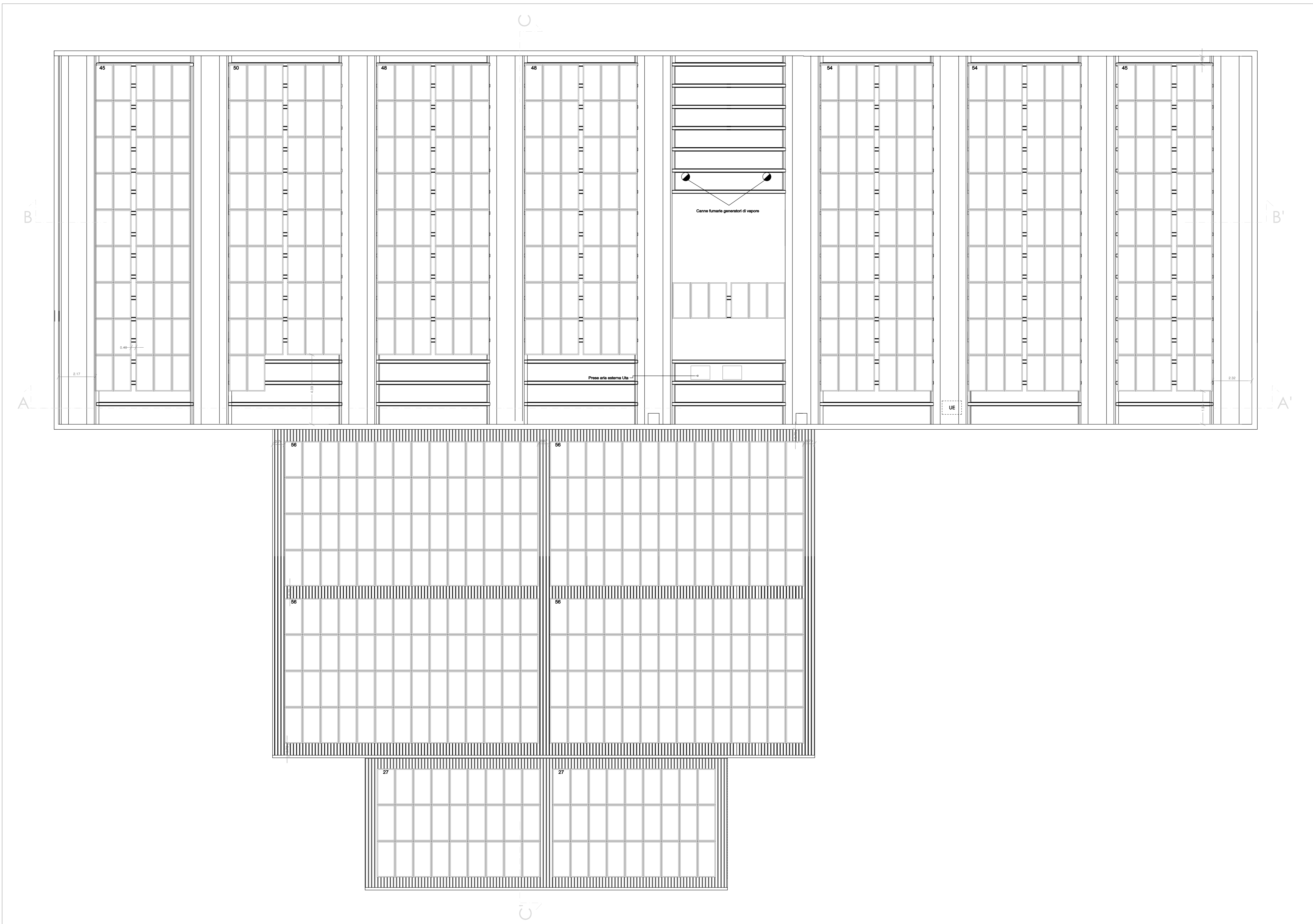
pianta copertura caseificio
